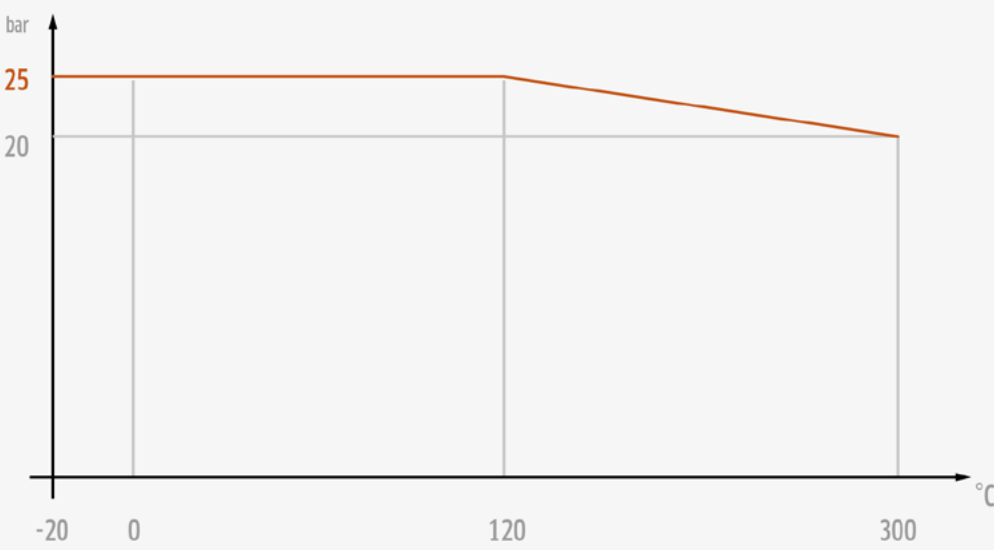
Wykres: relacja ciśnienie / temperatura
